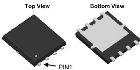
PDFN5x6-8L
